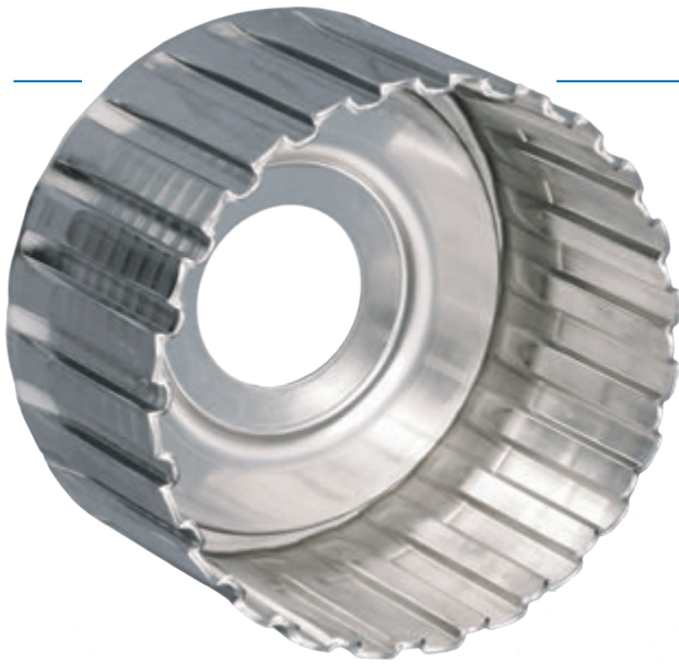
内歯、外歯スプライン付きクラッチディスクキャリアの冷間転造
