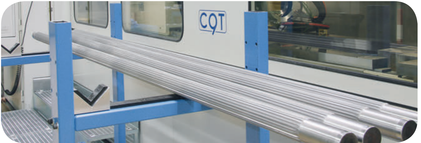
ツインスクリーュー押出機用スプラインシャフト
